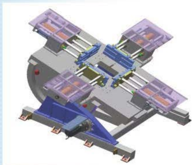
多功能浇铸机-30台
